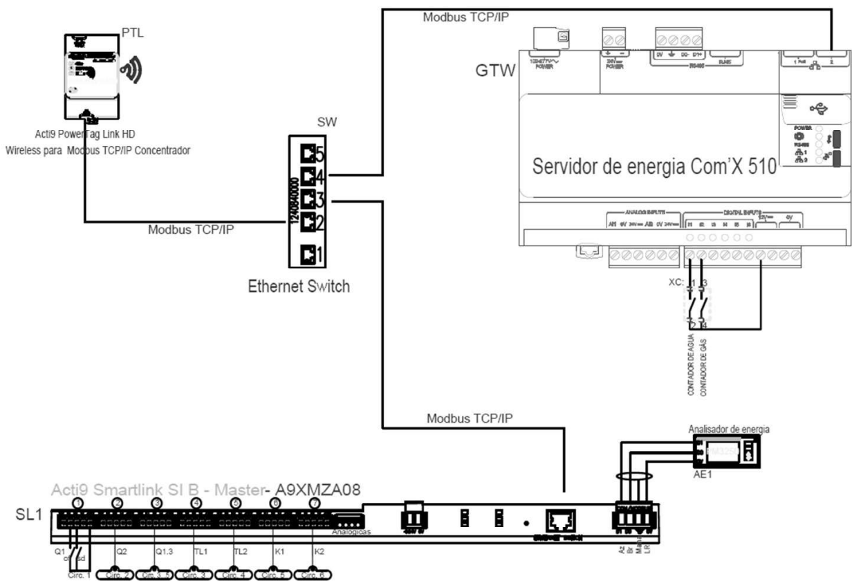
Figura 2. Esquema Unifilar de Comunicações
