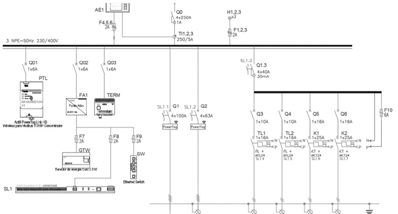
Figura 1. Esquema Unifilar de Potência
